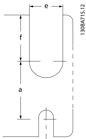
Илюстрация 8.3 Горни и долни монтажни отвори (B4, C3 и C4)
