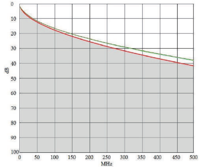
Attenuation
