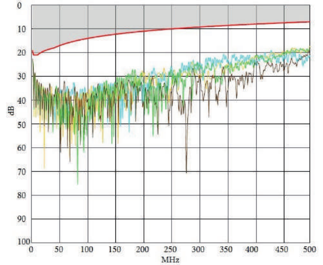
Attenuation
