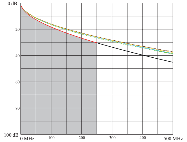
Attenuation
