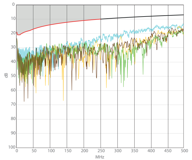
Attenuation
