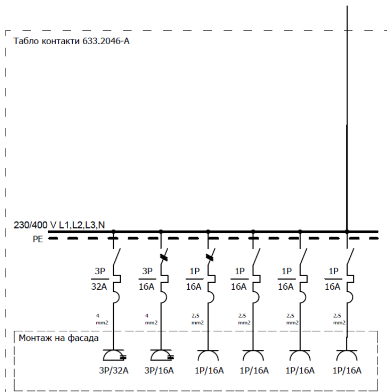
Табло контакти
